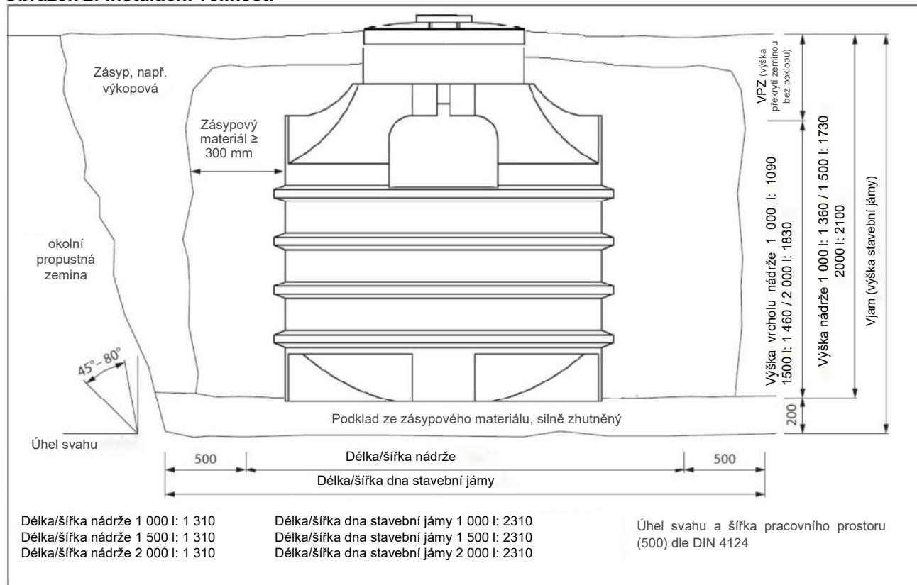
Obrázek 2: Instalační velikosti
