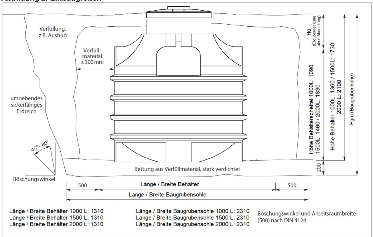
Abbildung 2: Einbaugrößen
