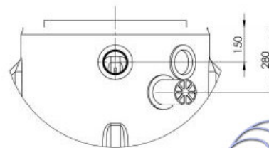
B (1 : 10)
