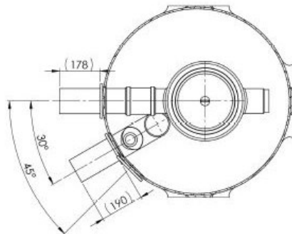
A-A (1 : 10)
