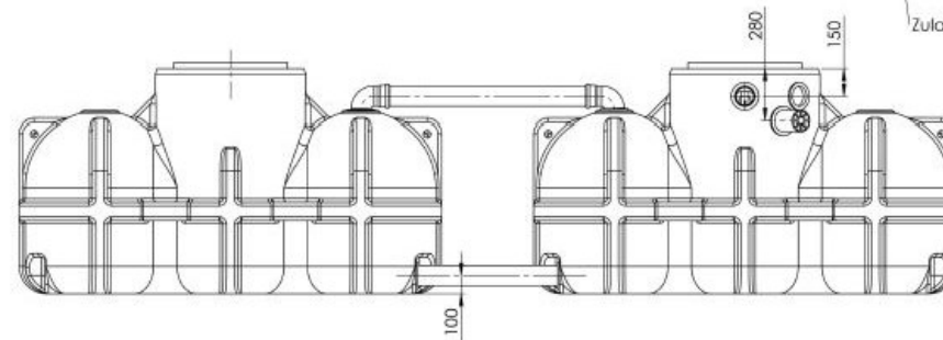
A-A (1 : 10)
