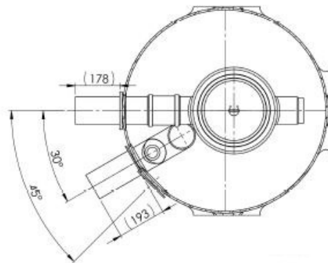
A-A (1 : 10)
