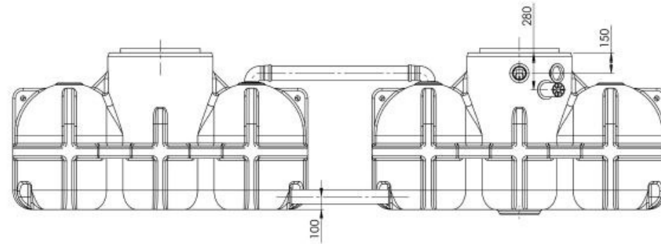
A-A (1 : 10)
