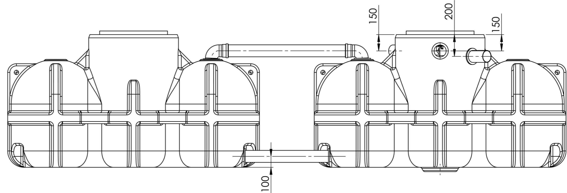
A-A (1 : 10)
