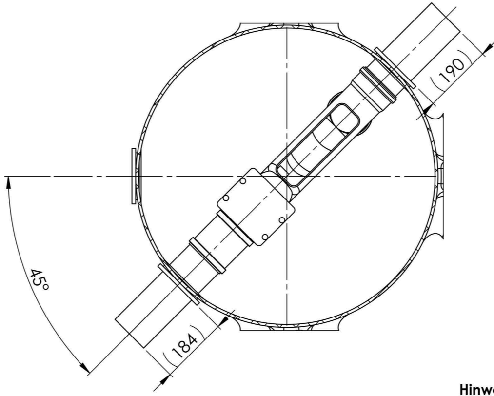
A-A (1 : 10)
