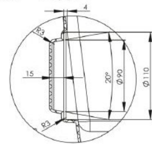
DETAIL D MAßSTAB 1 : 2
