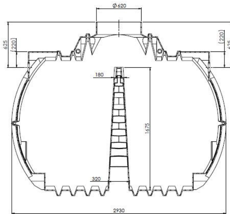
SCHNITT A-A
